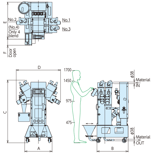
寸法図 Dimensions (mm)
